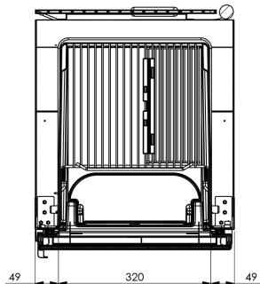
SEZIONE B-B
