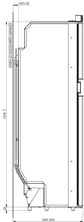
SEZIONE B-B
