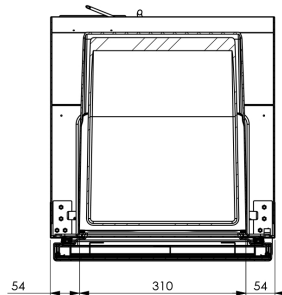
SEZIONE C-C
