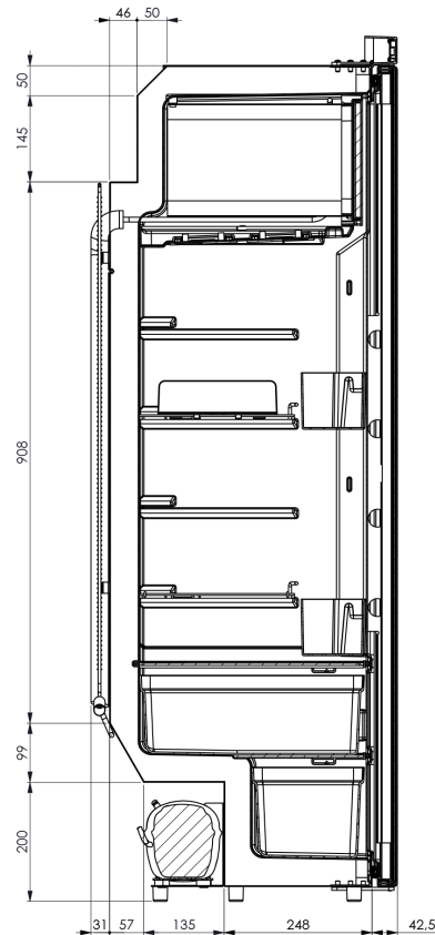
SEZIONE A-A
